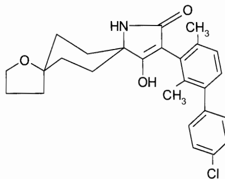
I-1-a-2
