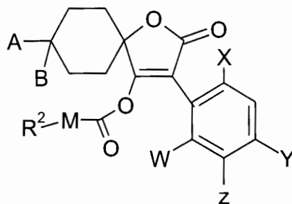
(I-2-c)
