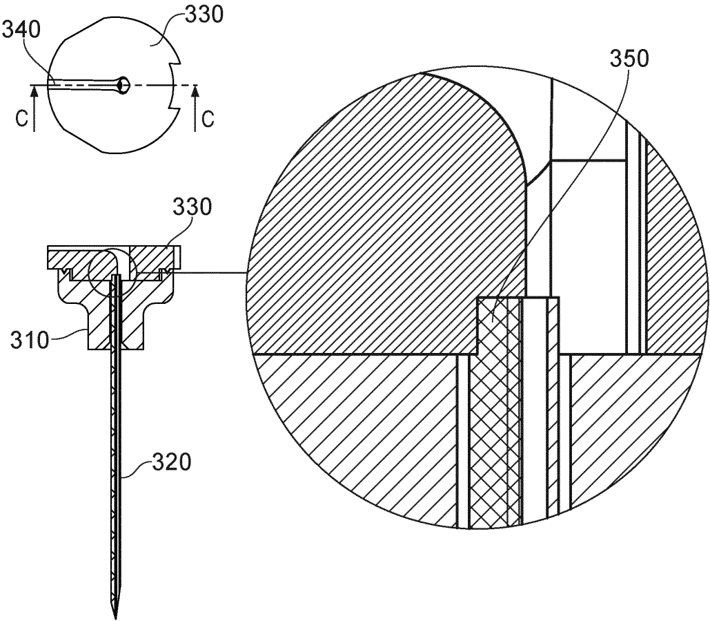
SECTION C-C FIG. 34(b)
