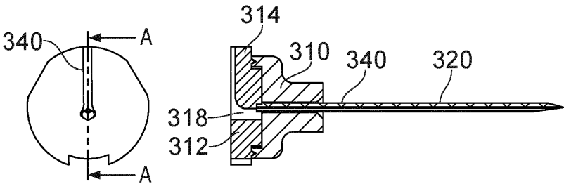
SECTION A-A FIG. 34(a)
