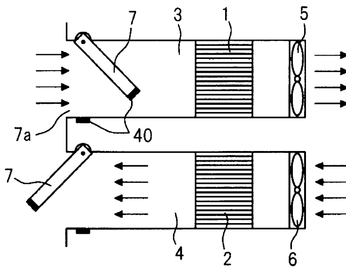
ドア開時(ファン動作)
