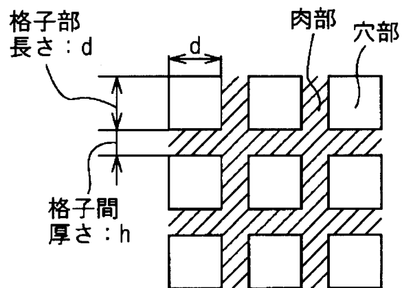
格子部拡大図
