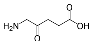
5-aminolevulinic acid (5-ALA)
