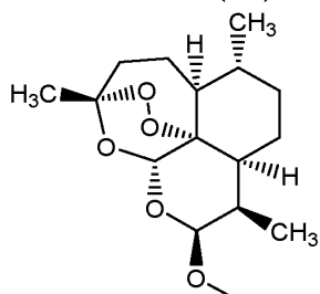
artemether ( 1c )
