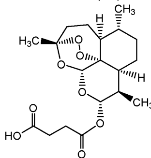
artesunate ( 1e )
