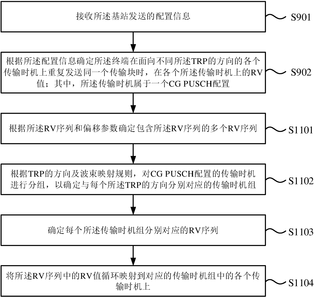
图 11
