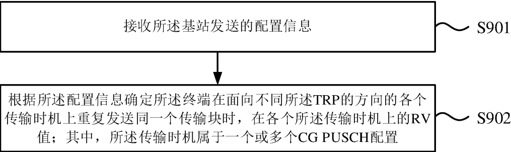
图 9
