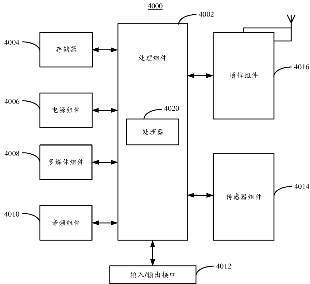
图 40
