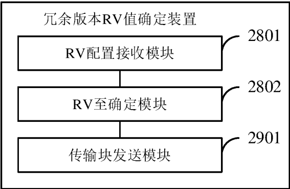
图 29
