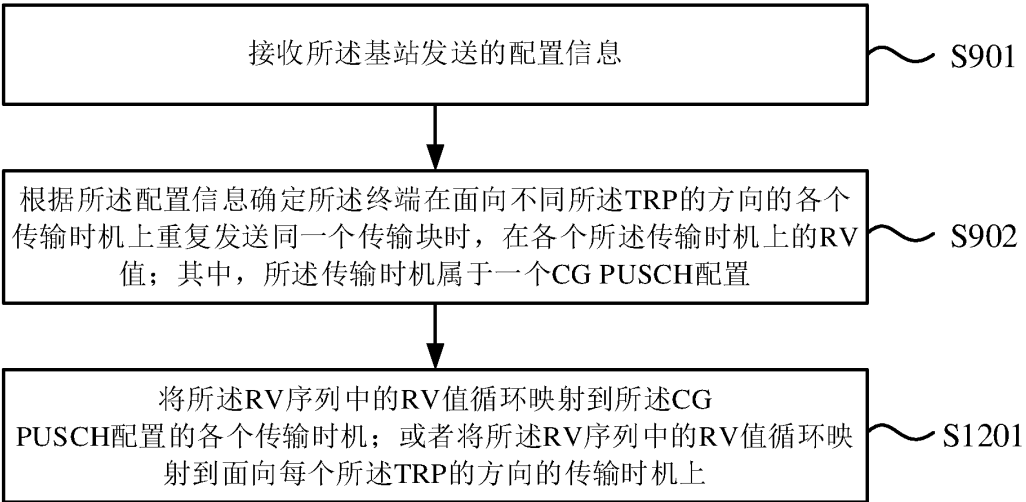
图 12
