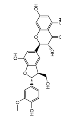
Silychristin
