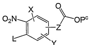
(A2)
