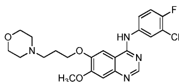
Gefitinib
