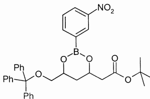
Formula VIId
