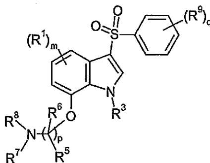
Ia2
