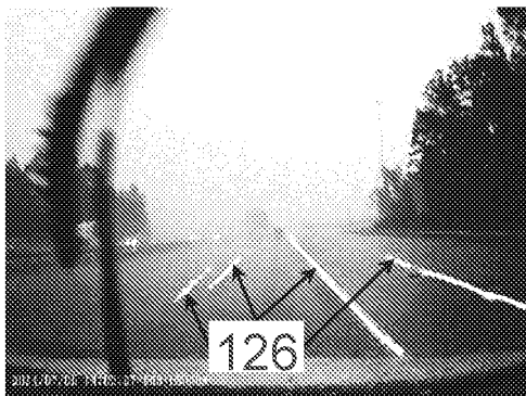
(d) lane enhancement by semi-supervised translation
