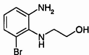
B. 2-[(2-amino-6-bromophenyl)amino]ethanol
