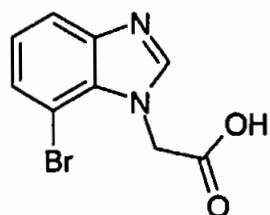
3)(7-Bromo-1H-benzimidazol-1-yl)acetic acid
