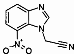
A. (7-Nitro-1H-benzimidazol-1-yl)acetonitrile
