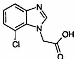
4)(7-Chloro-1H-benzimidazol-1-yl)acetic acid
