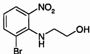
A. 2-[(2-bromo-6-nitrophenyl)amino]ethanol
