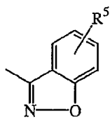
(b-10)
