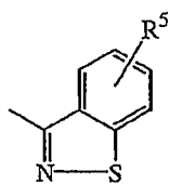
(b-9)
