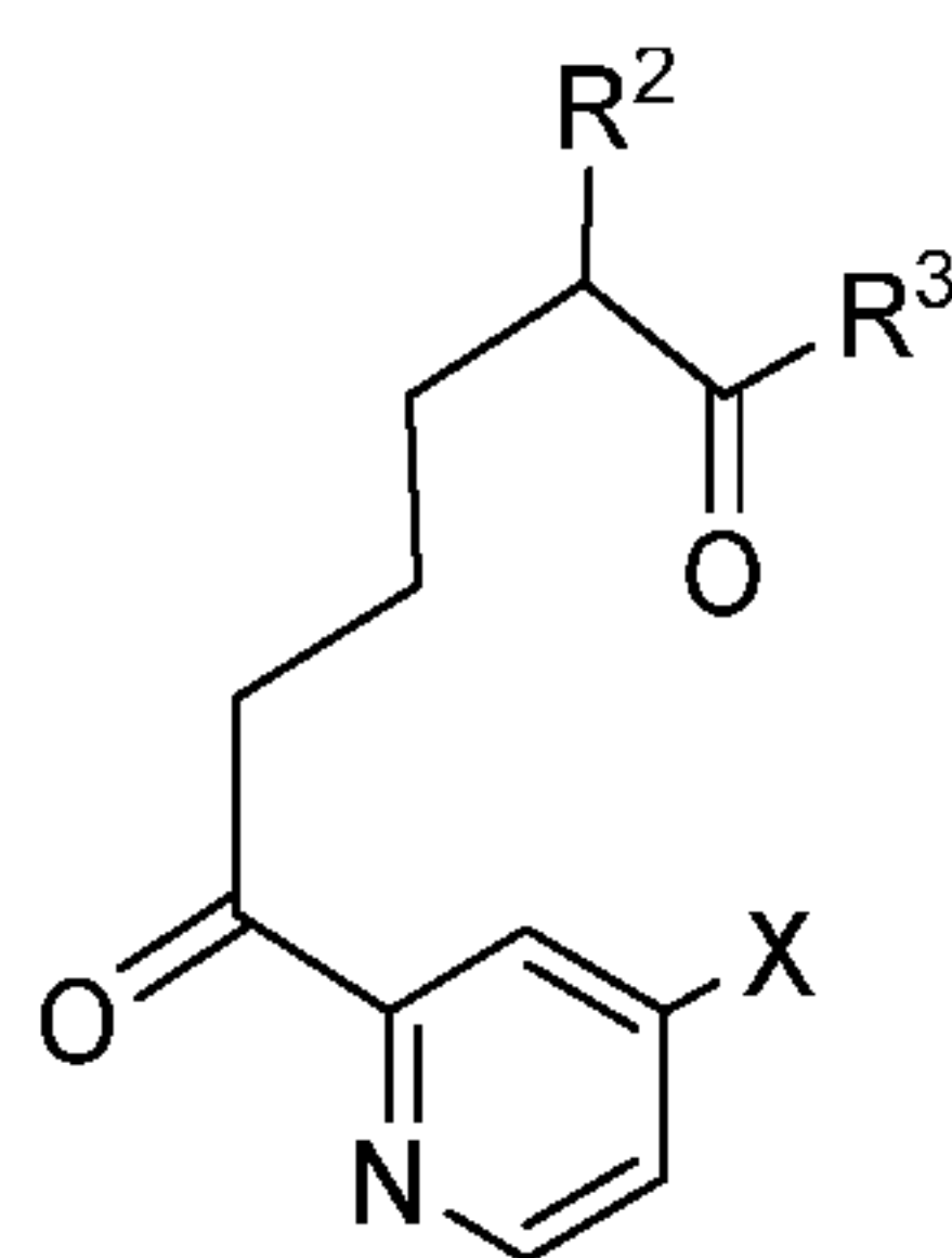
(VI)
