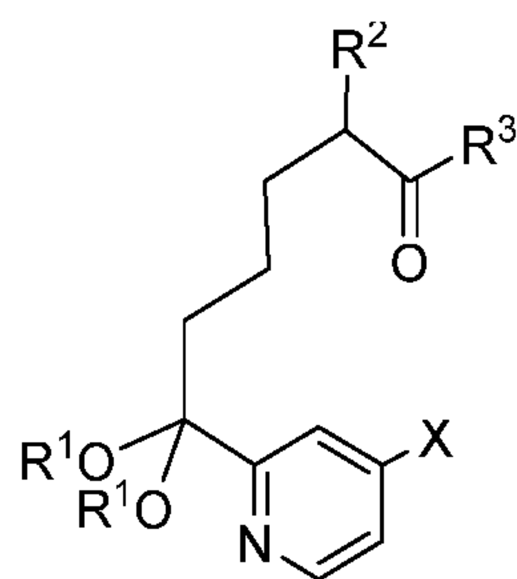
(II)
