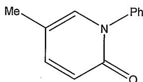
Pirfenidone analogs
