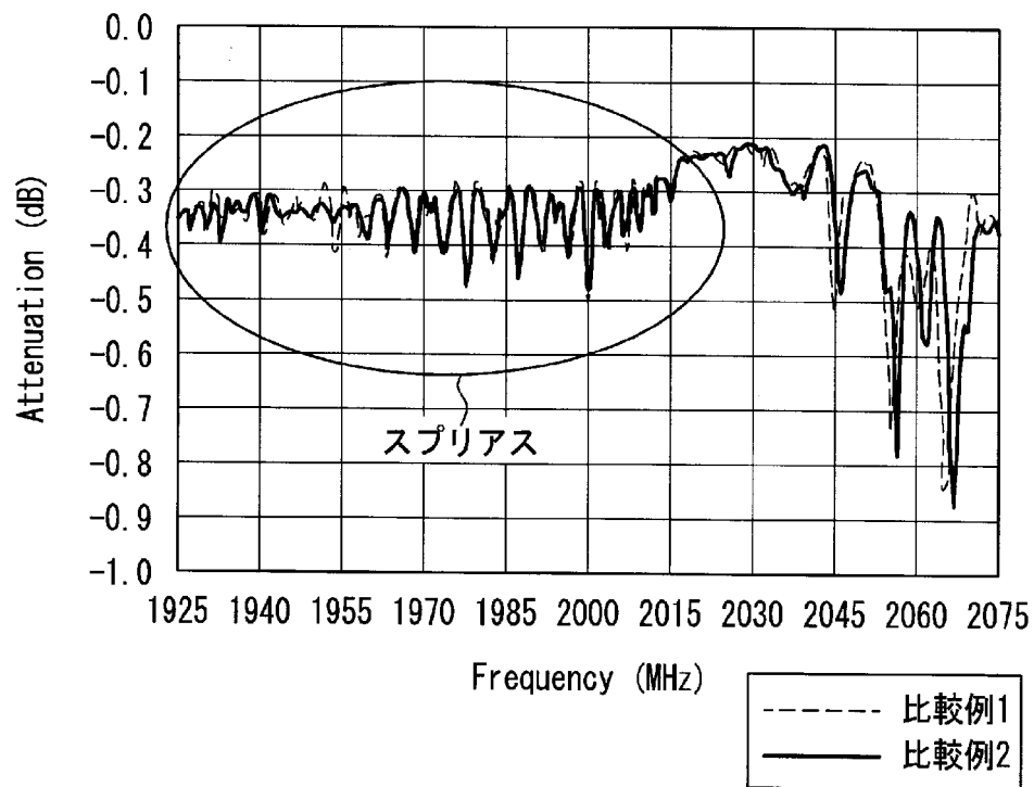
圧電薄膜共振子の共振特性
