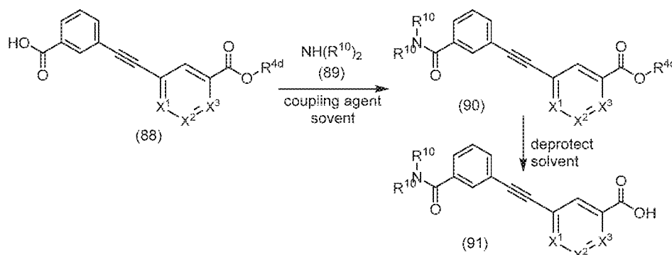
Scheme 20.
