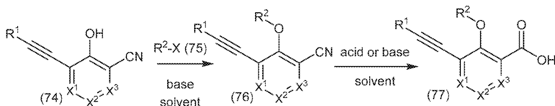
Scheme 17.
