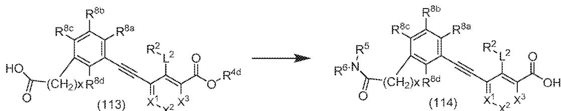
Scheme 27.
