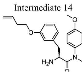
(S)-2-amino-3-(3-(but-3-en-1-yloxy)phenyl)-N-(4-methoxyphenyl)-N-methylpropanamide
