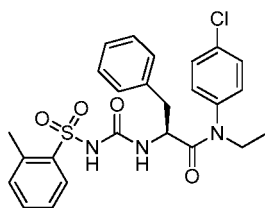
(S) -N-(4-chlorophenyl)-N-ethyl-3-phenyl-2-(3-(o-tolylsulfonyl)ureido)propanamide
