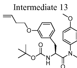
(S)-tert-butyl (3-(3-(but-3-en-1-yloxy)phenyl)-1-((4-methoxyphenyl)(methyl)amino)-1-oxopropan-2-yl)carbamate
