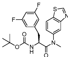
(S)-tert-butyl (1-(benzo[d]thiazol-5-yl(methyl)amino)-3-(3,5-difluorophenyl)-1-oxopropan-2-yl)carbamate
