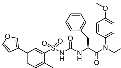
(S)-N-ethyl-2-(3-((5-(furan-3-yl)-2-methylphenyl)sulfonyl)ureido)-N-(4-methoxyphenyl)-3-phenylpropanamide
