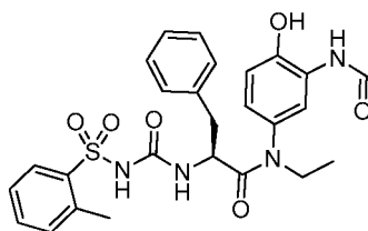
(S)-N-ethyl-N-(3-formamido-4-hydroxyphenyl)-3-phenyl-2-(3-(o-tolylsulfonyl)ureido)propanamide
