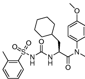
(S)-3-cyclohexyl-N-(4-methoxyphenyl)-N-methyl-2-(3-(o-tolylsulfonyl)ureido)propanamide
