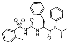
(S)-N-isopropyl-N,3-diphenyl-2-(3-(o-tolylsulfonyl)ureido)propanamide
