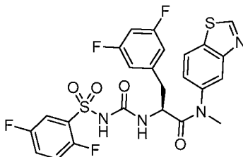
(S)-N-(benzo[d]thiazol-5-yl)-3-(3,5-difluorophenyl)-2-(3-((2,5-difluorophenyl)sulfonyl)ureido)-N-methylpropanamide
