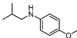
N-isobutyl-4-methoxyaniline
