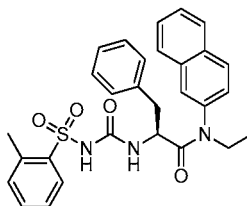
(S)-N-ethyl-N-(naphthalen-2-yl)-3-phenyl-2-(3-(o-tolylsulfonyl)ureido)propanamide
