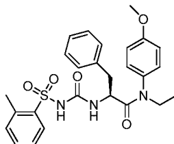
(S)-N-ethyl-N-(4-methoxyphenyl)-3-phenyl-2-(3-(o-tolylsulfonyl)ureido)propanamide
