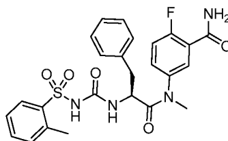
(S)-2-fluoro-5-(N-methyl-3-phenyl-2-(3-(o-tolylsulfonyl)ureido)propanamido)benzamide
