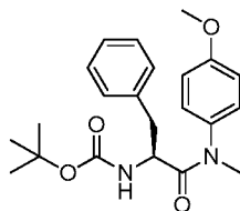
(S)-tert-butyl (1-((4-methoxyphenyl)(methyl)amino)-1-oxo-3-phenylpropan-2-yl)carbamate
