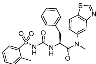
(S)-N-(benzo[d]thiazol-5-yl)-N-methyl-3-phenyl-2-(3-(o-tolylsulfonyl)ureido)propanamide
