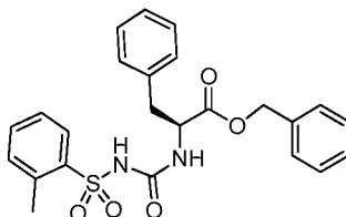
(S)-benzyl 3-phenyl-2-(3-(o-tolylsulfonyl)ureido)propanoate
