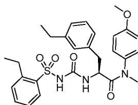
(S)-3-(3-ethylphenyl)-2-(3-((2-ethylphenyl)sulfonyl)ureido)-N-(4-methoxyphenyl)-N-methylpropanamide
