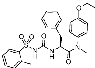
(S)-N-(4-ethoxyphenyl)-N-methyl-3-phenyl-2-(3-(o-tolylsulfonyl)ureido)propanamide
