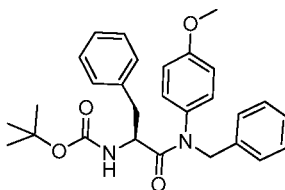
(S)-tert-butyl (1-(benzyl(4-methoxyphenyl)amino)-1-oxo-3-phenylpropan-2-yl)carbamate
