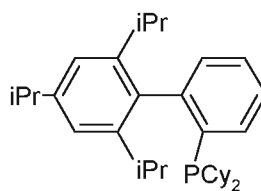
XPhos
