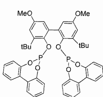
biphephos
