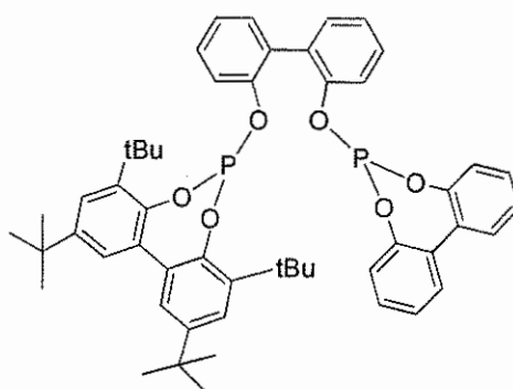
ligand (91a)
