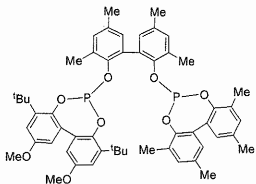
ligand (11a)
