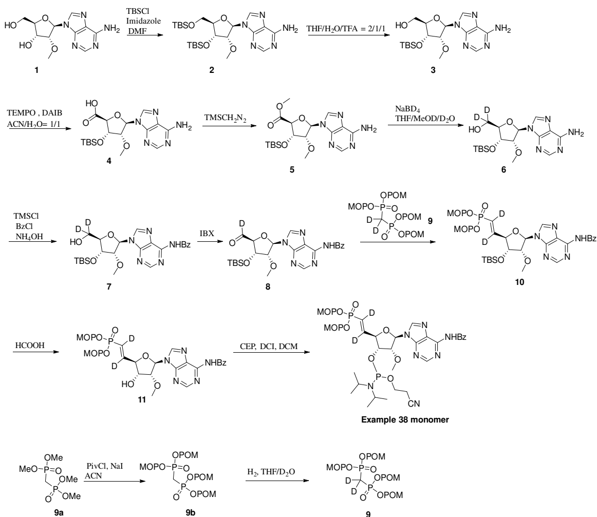
Scheme-18
