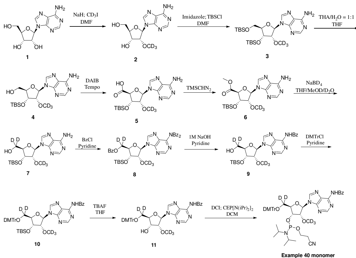
Scheme-20
