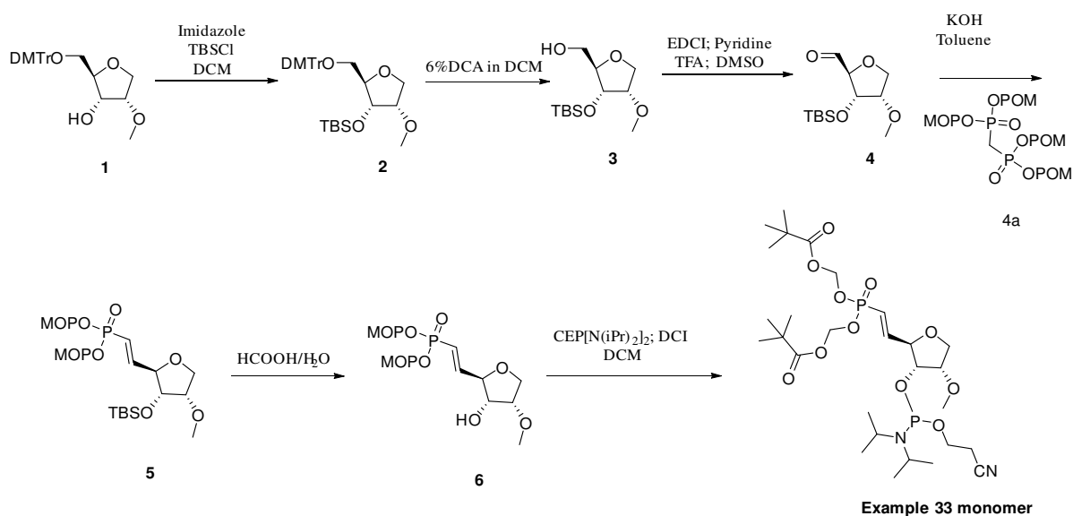
Scheme-13
