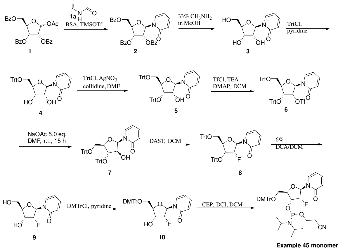
Scheme-25
