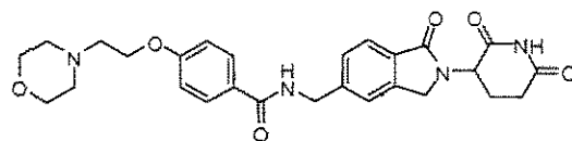
N-((2-(2,6-dioxopiperidin-3-yl)-1-oxoisoindolin-5-yl)methyl)-4-(2-morpholinoethoxy)benzamide;
