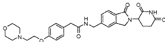
N-((2-(2,6-dioxopiperidin-3-yl)-1-oxoisindolin-5-yl)methyl)-2-(4-(2-morpholinoethoxy)phenyl)acetamide;
