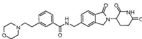
N-((2-(2,6-dioxopiperidin-3-yl)-1-oxoisoindolin-5-yl)methyl)-3-(2-morpholinoethyl)benzamide;
