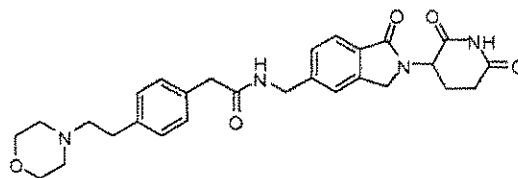
N-((2-(2,6-dioxopiperidin-3-yl)-1-oxoisindolin-5-yl)methyl)-2-(4-(2-morpholinoethyl)phenyl)acetamide;
