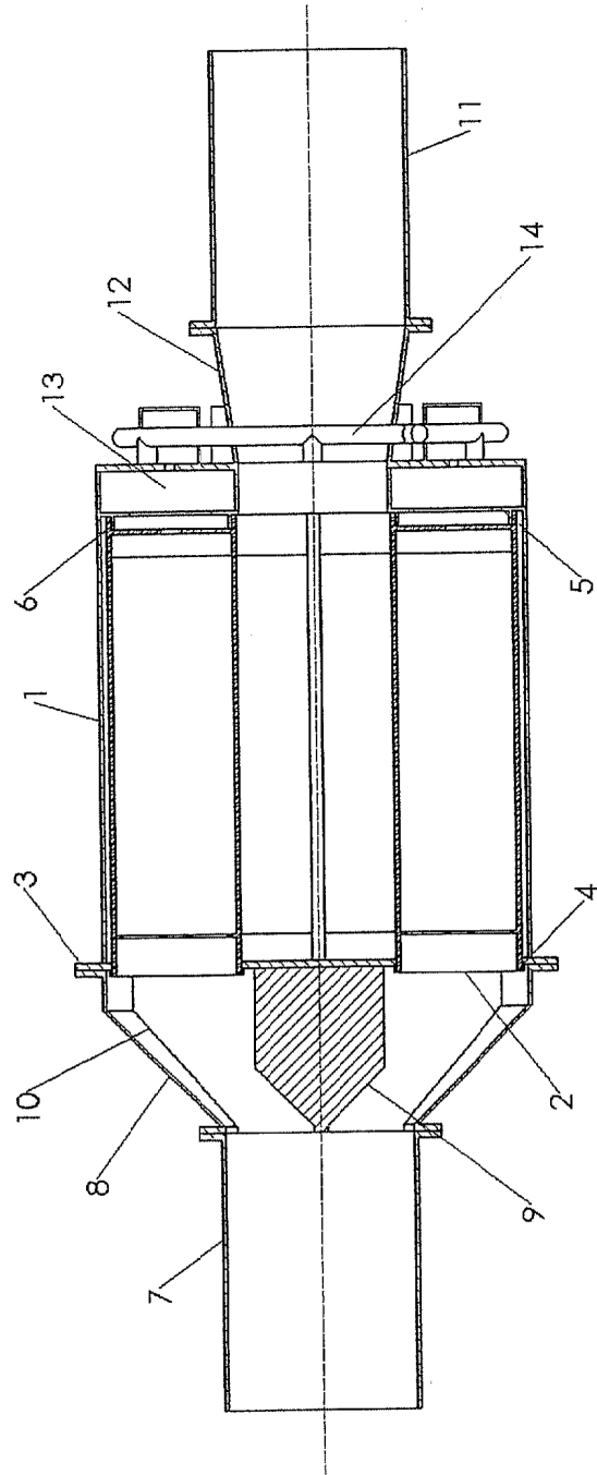
SECTION A-A
