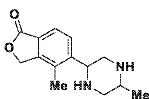
Enantiomer-I (153-I)
