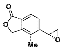
Enantiomer-I (1-I)
