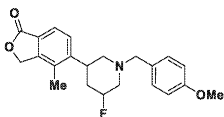
Enantiomer-I (122G-I)
