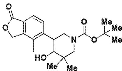
Enantiomer-I (73B-I)
