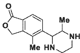
Enantiomer-I (71-I)
