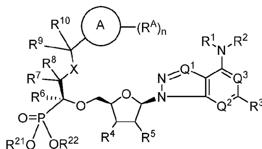
Formula (Ia).
