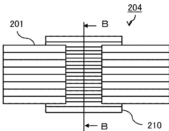
A拡大図
