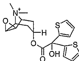
Tiotropium
