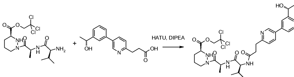
Compound 44e
