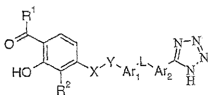
tautomer I
