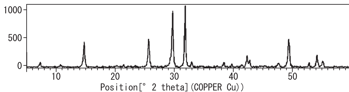
FIG. 1B
