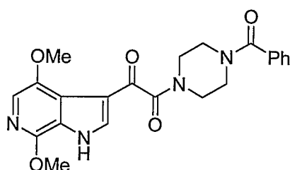
IVa
