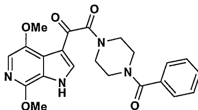
IVa
