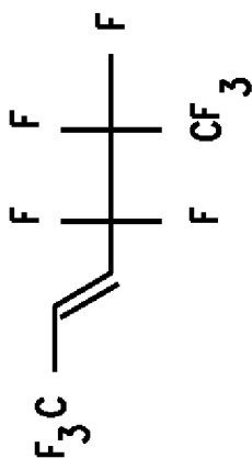
(2E)-1,1,1,4,4,5,5,6,6,6-decafluorohex-2-ene
