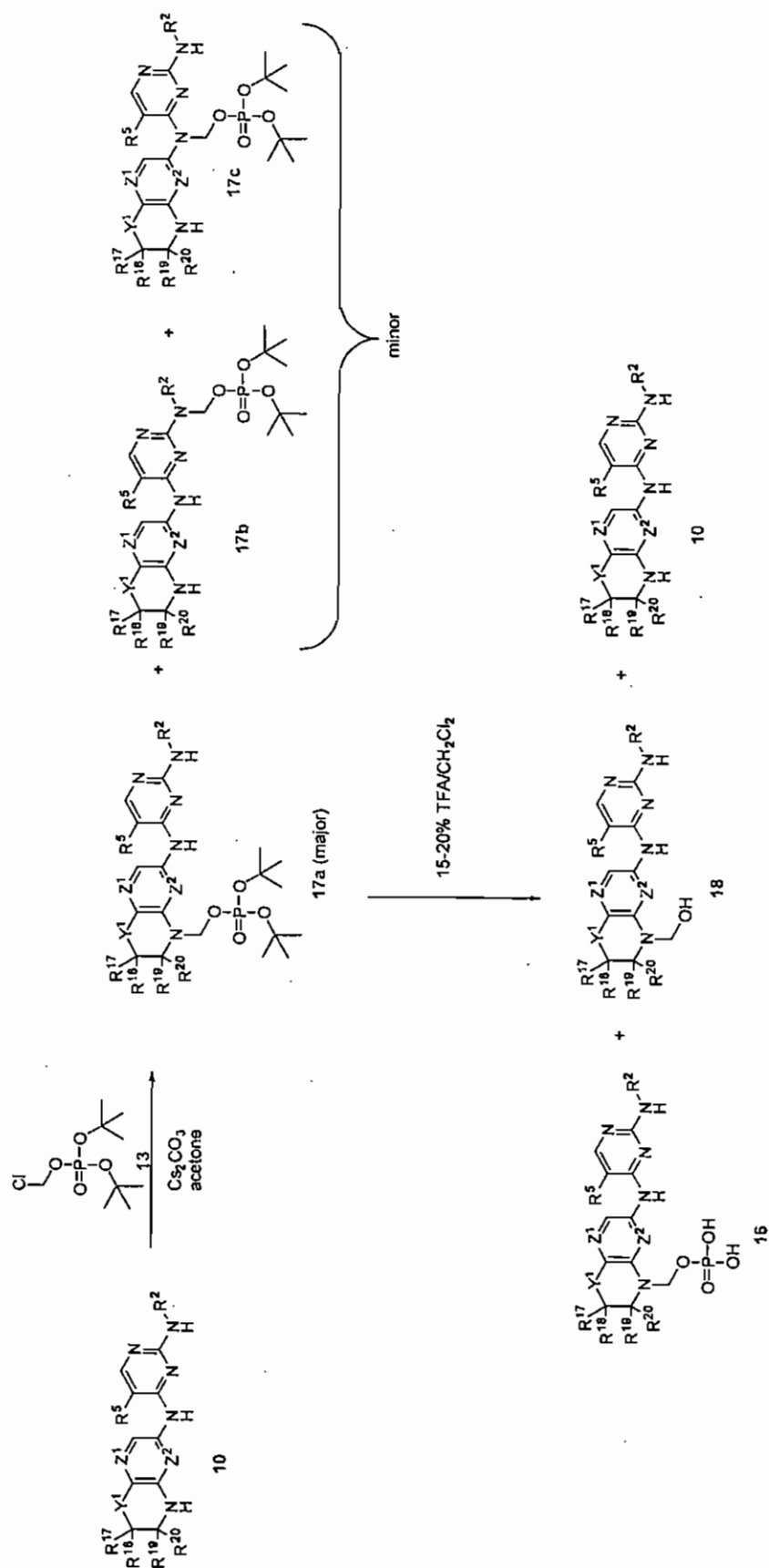
Scheme (IV)
