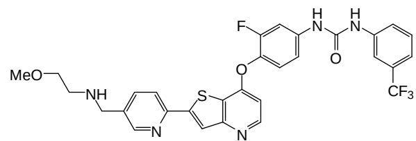
(Cpd. 271, example 164).
