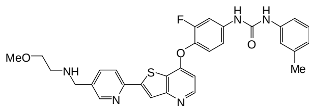
(Cpd. 268, example 161).
