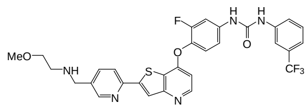
(Cpd. 271, example 164),
