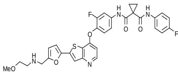
(Cpd. 254, example 147).
