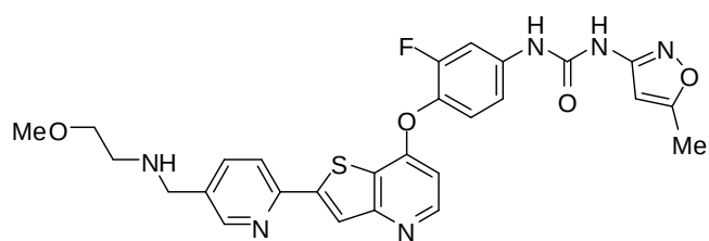
(Cpd. 149, example 53).
