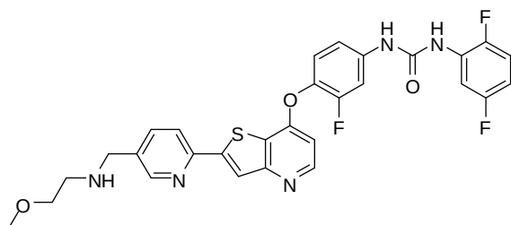
(Cpd. 337, example 223).
