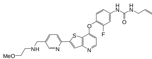
(Cpd. 274, example 167).
