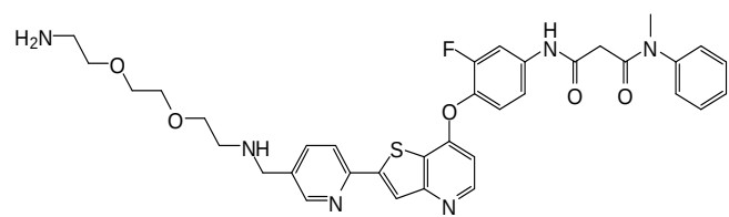
(Cpd. 293, example 183).
