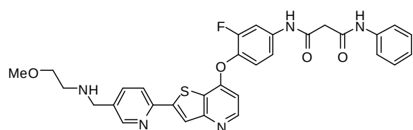
(Cpd. 235, example 128).
