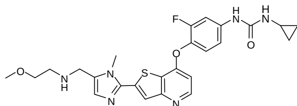
(Cpd. 341 example 227).
