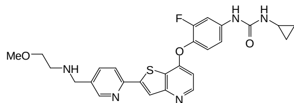
(Cpd. 277, example 170).
