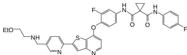
(Cpd. 281, example 174),
