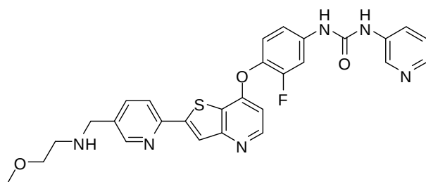
(Cpd. 354 example 240).
