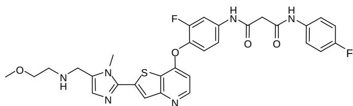
(Cpd. 343 example 229).
