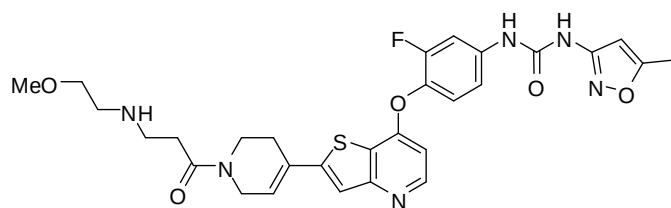
(Cpd. 351 example 237),
