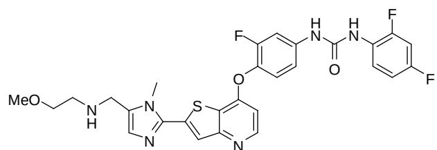
(Cpd. 359 example 245).
