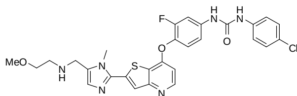
(Cpd. 368 example 254).
