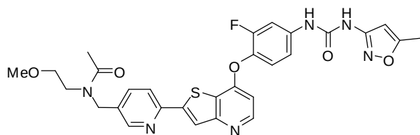
(Cpd. 339 example 225).
