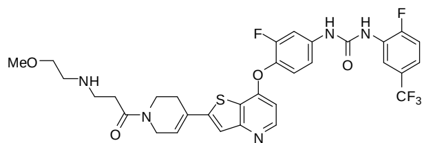
(Cpd. 353 example 239).
