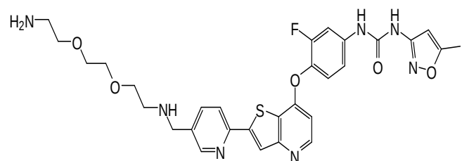
(Cpd. 294, example 184).
