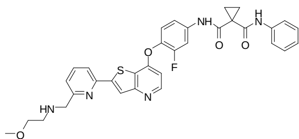
(Cpd. 224, example 117).
