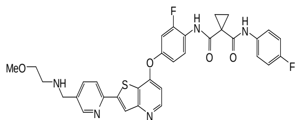
(Cpd. 273, example 166).
