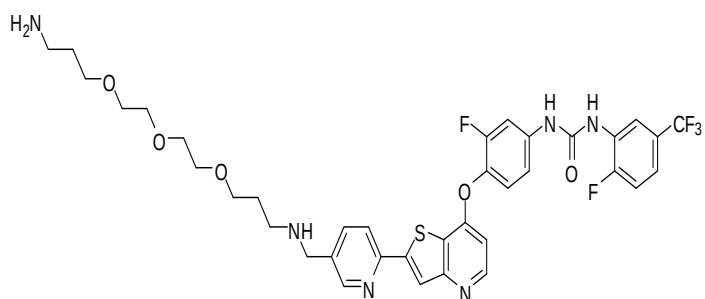
(Cpd. 284, example 177).
