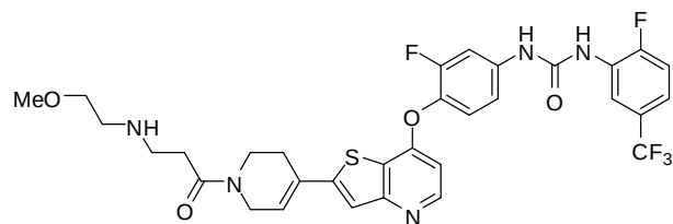
(Cpd. 353 example 239).
