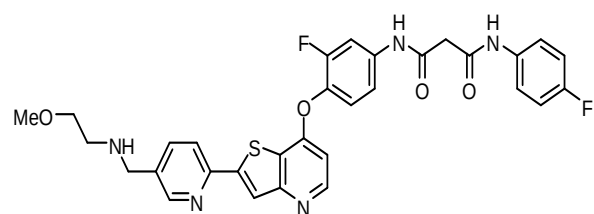
(Cpd. 237, example 130).
