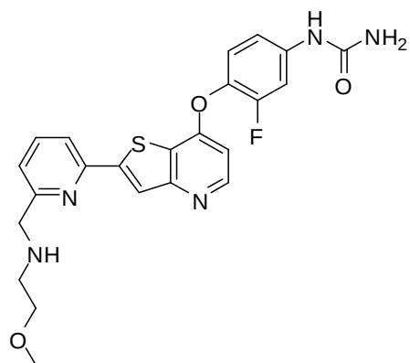
(Cpd. 318, example 204).
