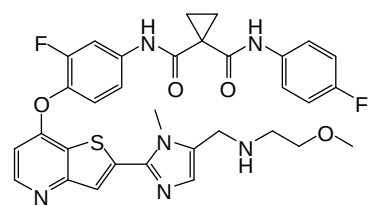
(Cpd. 270, example 163).
