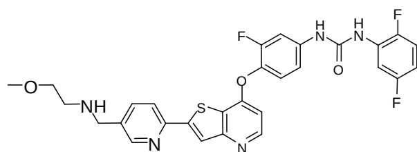
(Cpd. 349 example 235).
