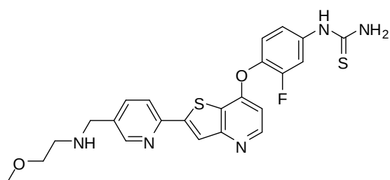
(Cpd. 319, example 205).
