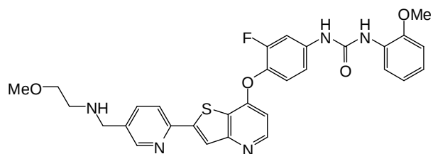
(Cpd. 267, example 160).
