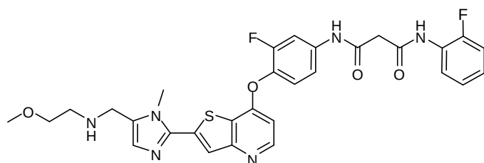
(Cpd. 342 example 228).
