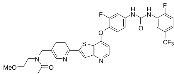
(Cpd. 355 example 241).
