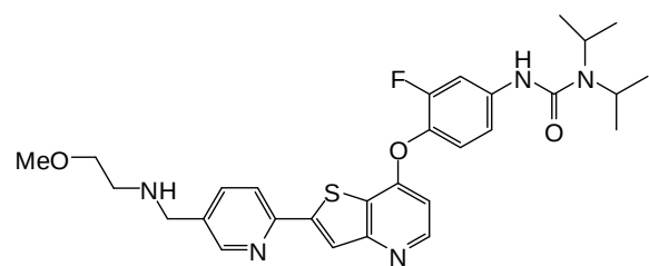
(Cpd. 261, example 154).
