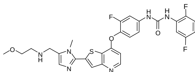
(Cpd. 347 example 233).
