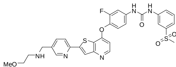
(Cpd. 336, example 222).
