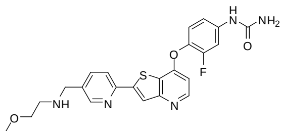
(Cpd. 289, example 180).
