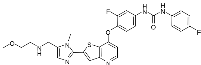
(Cpd. 346 example 232).
