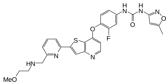
(Cpd. 269, example 162).
