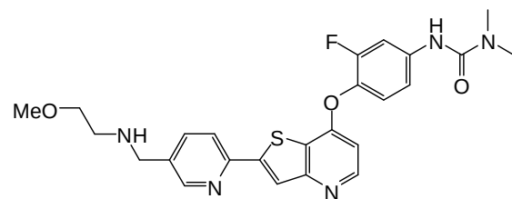
(Cpd. 272, example 165).
