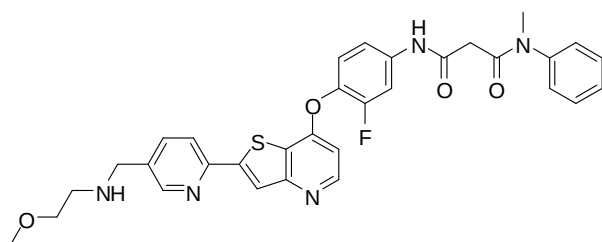
(Cpd. 223, example 116).
