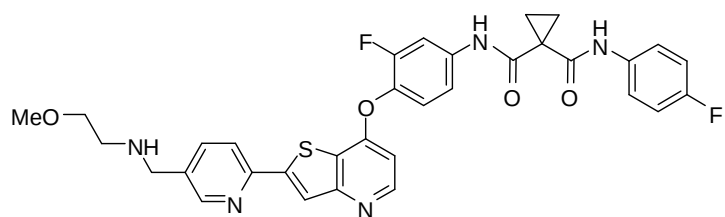
(Cpd. 147, example 52).
