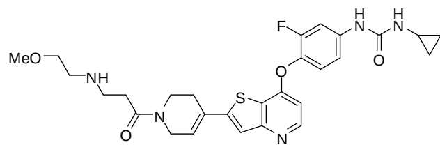
(Cpd. 352 example 238).
