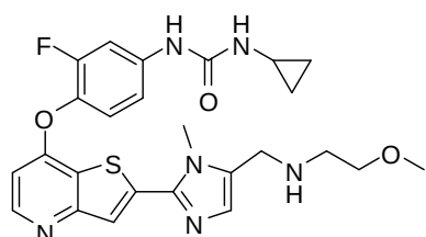
(Cpd. 287, example 179).
