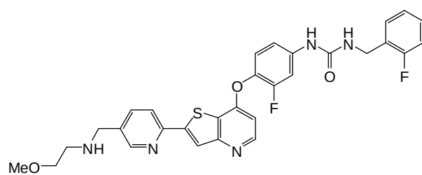
(Cpd. 275, example 168).
