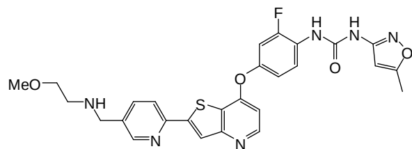
(Cpd. 259, example 152).
