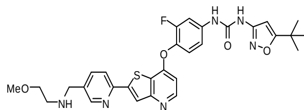
(Cpd. 252, example 145).
