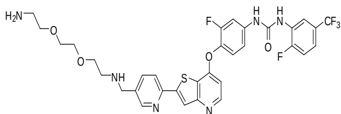
(Cpd. 285, example 178).
