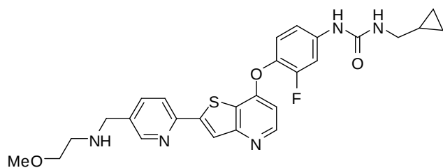
(Cpd. 358 example 244).
