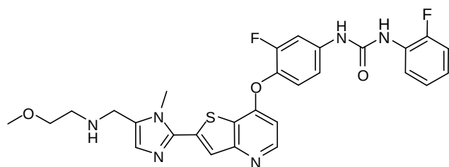
(Cpd. 345 example 231).
