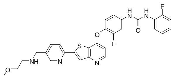
(Cpd. 332, example 218).
