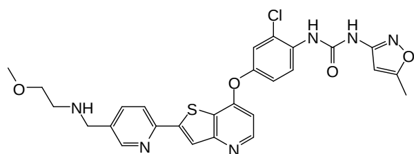
(Cpd. 298a, example 188a).
