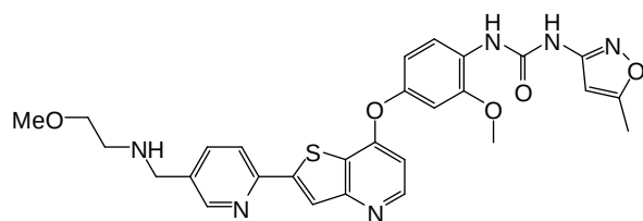
(Cpd. 262, example 155).
