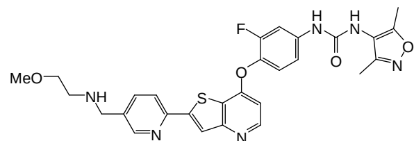
(Cpd. 266, example 159).
