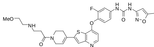
(Cpd. 351 example 237).
