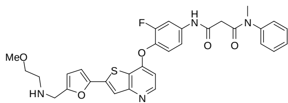
(Cpd. 283, example 176).
