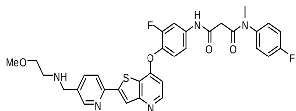
(Cpd. 236, example 129).
