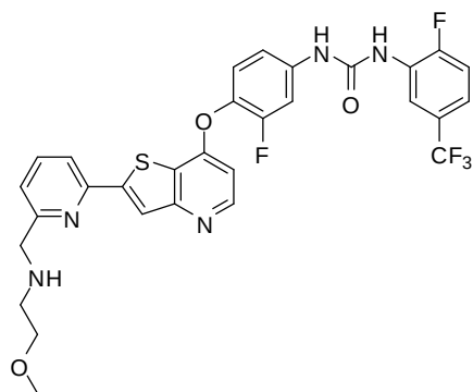
(Cpd. 322, example 208).
