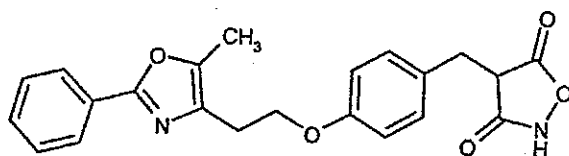
JTT-501
