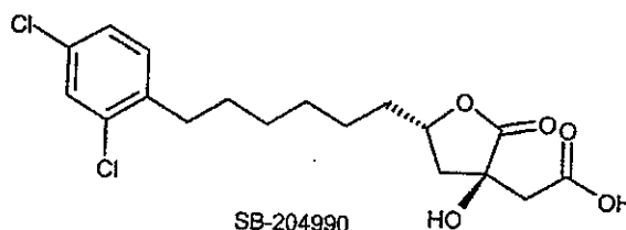
SB-204990
