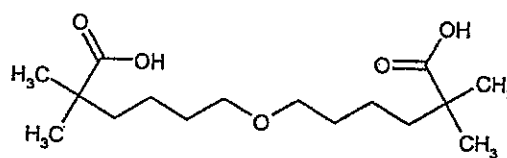
CI-1027
