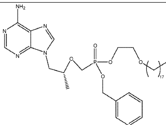
Octadecyloxyethyl benzyl tenofovir (ODE-Bn-TFV)
