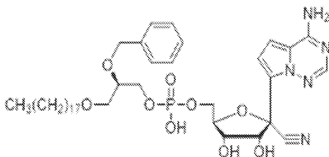
1-O-octadecyl-2-O-benzyl- sn -glyceryl-phospho-RVn
