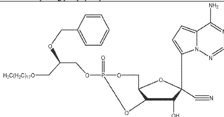
1- O -octadecyl- sn -glyceryl- phospho -RVn
