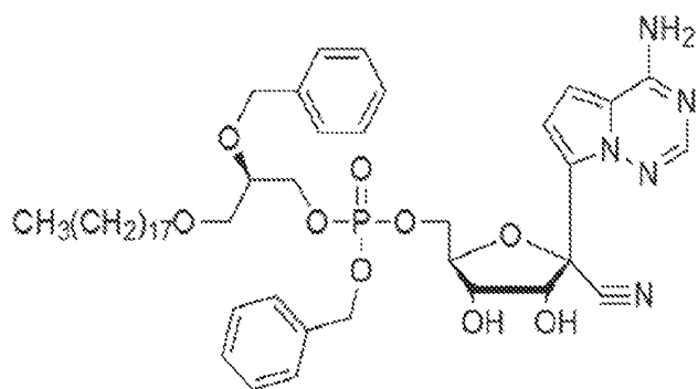
1-O-octadecyl-2-O-benzyl- sn -glyceryl-benzyl-phospho-RVn
