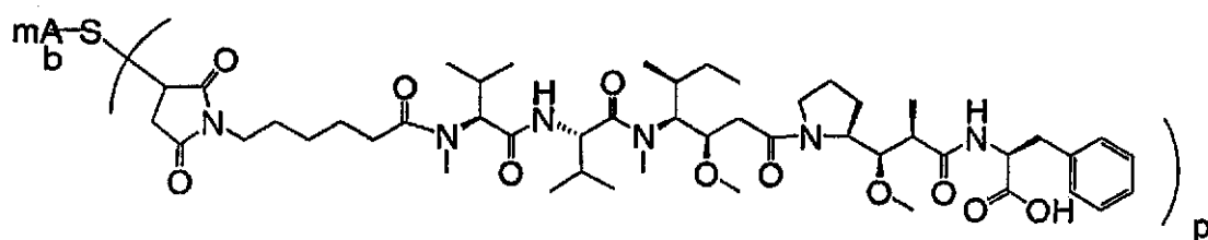
L-MC-MMAF
