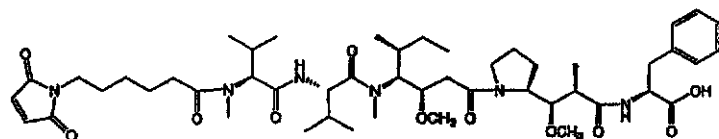
MC-MMAF
