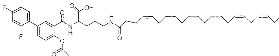
IVb-7
