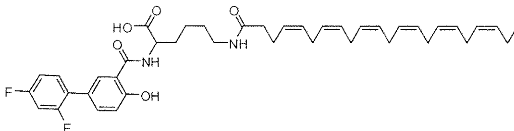
IVc-5
