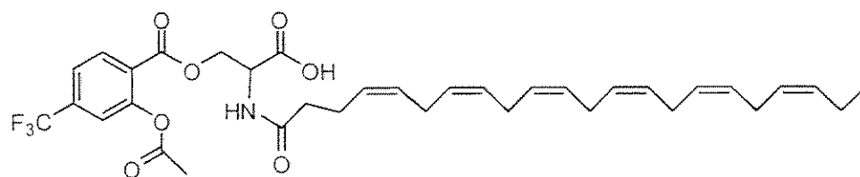
VIb-10
