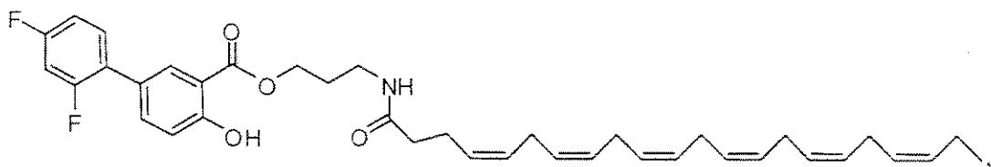
IVc-3
