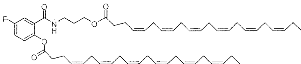
Id-3
