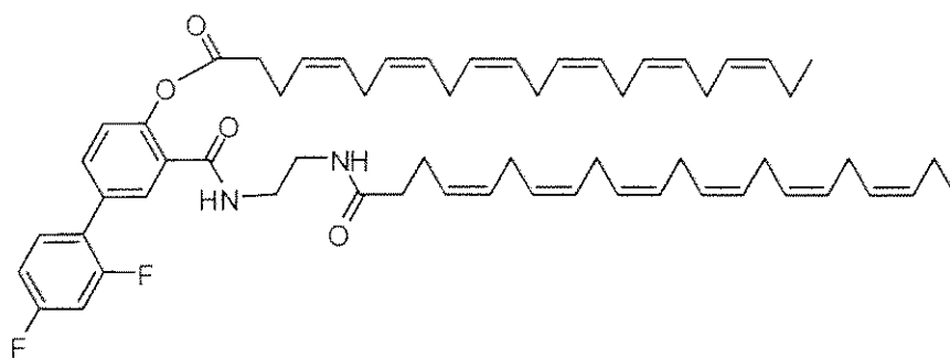
IVc-7
