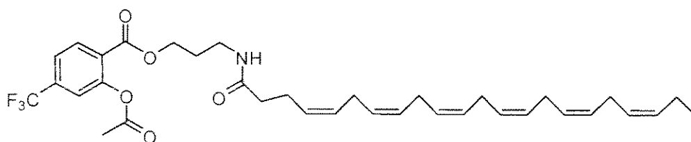
VIb-2
