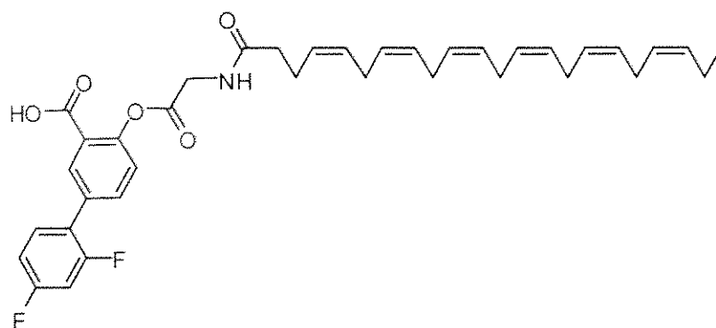
IVf-1
