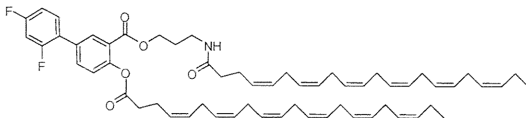
IVc-5
