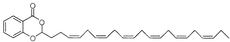
If-2
