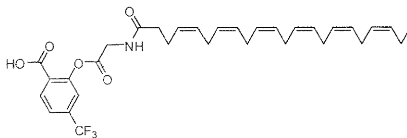
VIg-3
