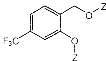
Formula VIId
