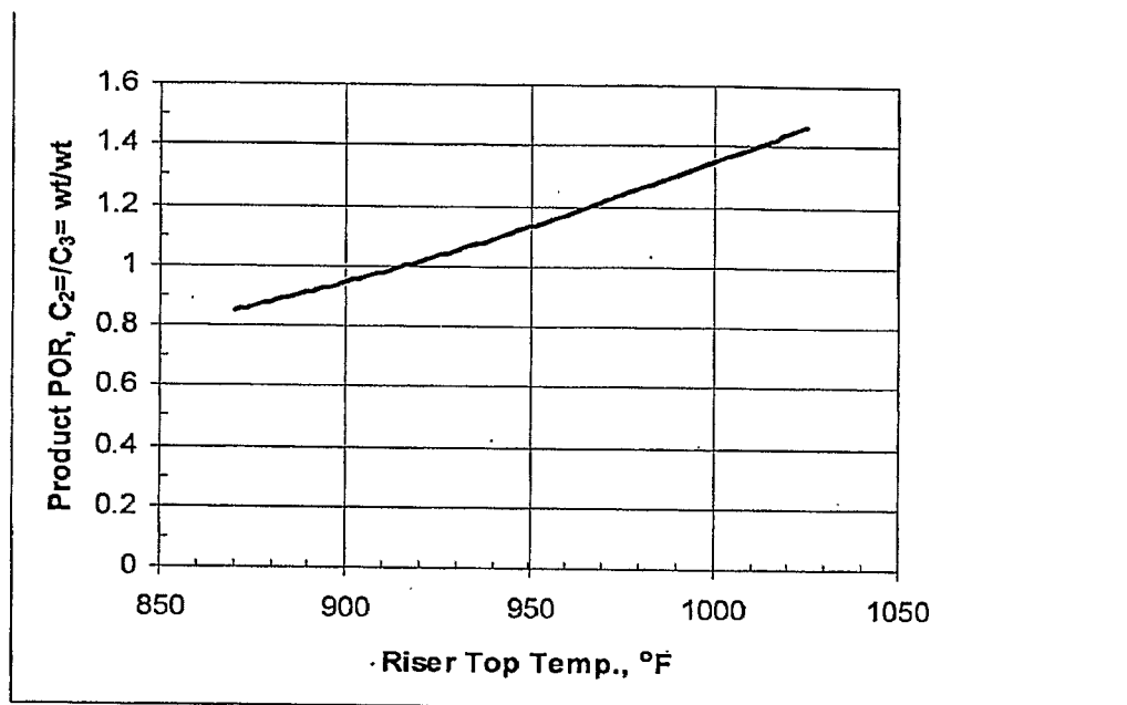
Predicted POR versus Riser Top Temperature
