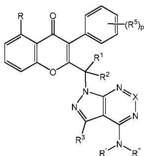
(IA-VI)
