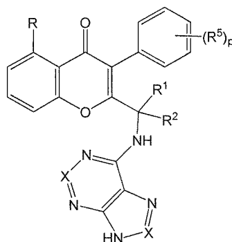
(IA-VIII)
