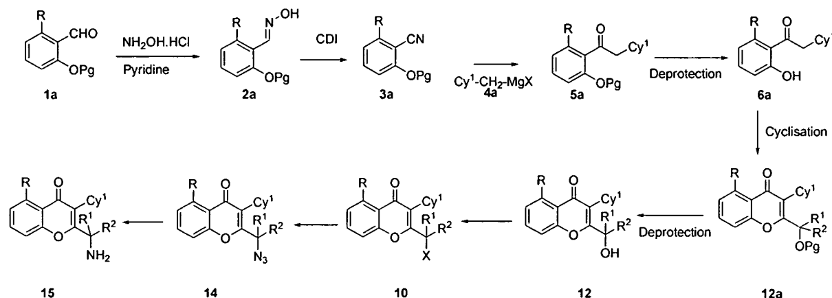
SCHEME 1A
