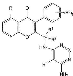
(IA-VII)
