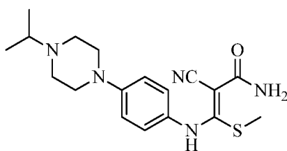
2-cyano-3-((4-(4-isopropylpiperazin-1-yl)phenyl)amino)-3-(methylthio)acrylamide A1
