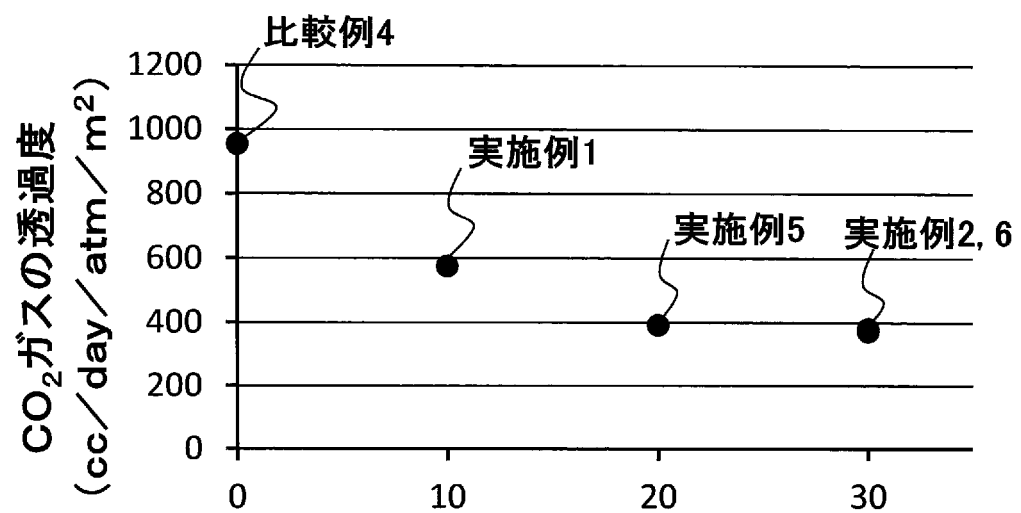
非晶性ポリアミド樹脂の配合割合(質量%)
