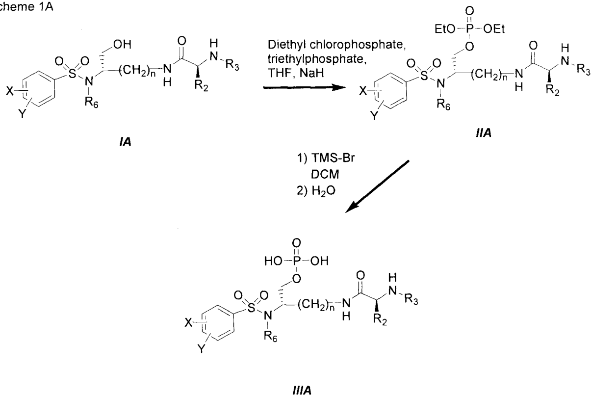
Scheme 1A
