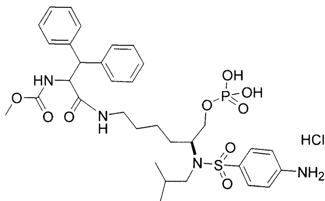
III B
