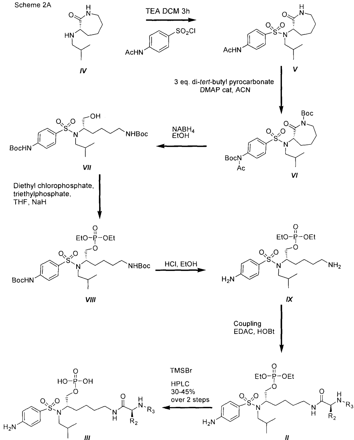
Scheme 2A
