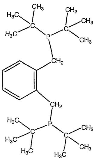
1,2-bis-(di-tert-butylphosphinomethyl)benzene
