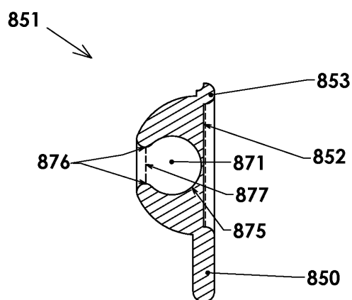
SECTION C-C FIG. 19F
