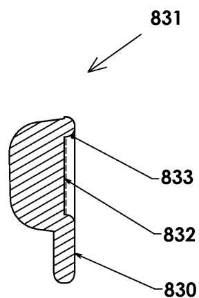
SECTION B-B FIG. 19E
