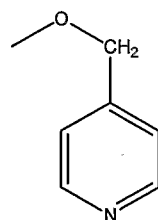
(4-picolyloxy)
