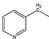
(3-picolyl)
