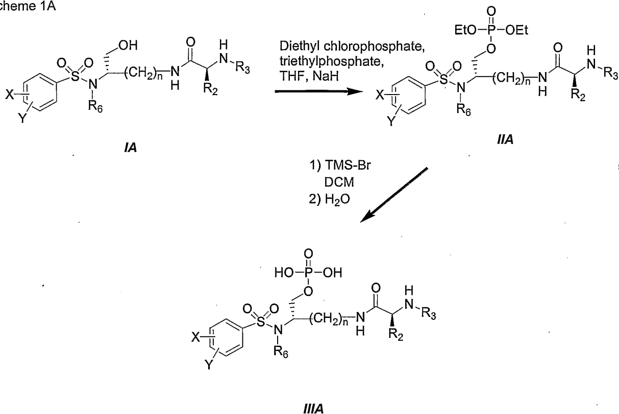
Scheme 1A
