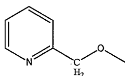
(2-picolyloxy)
