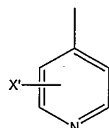
(substituted 4-pyridyl)
