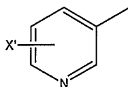
(substituted 3-pyridyl)
