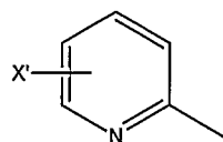
(substituted 2-pyridyl)
