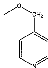
(4-picolyloxy)
