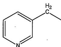
(3-picolyl)
