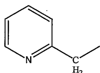
(2-picolyl)
