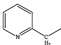
(2-picolyl)
