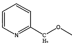
(2-picolyloxy)
