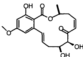
F152
