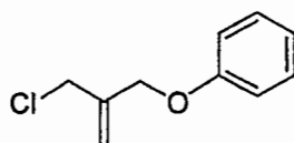
5-B (2-Chloromethyl-allyloxy)-benzene
