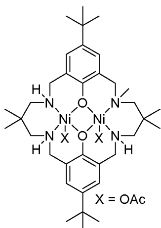
L^1Ni_2(OAc)_2
