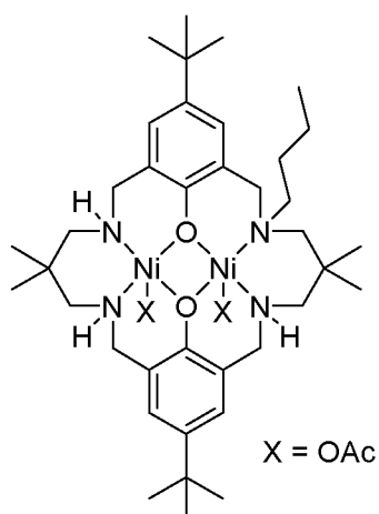
L^4Ni_2(OAc)_2
