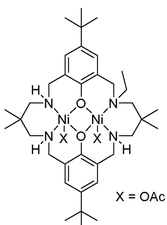
L^2Ni_2(OAc)_2
