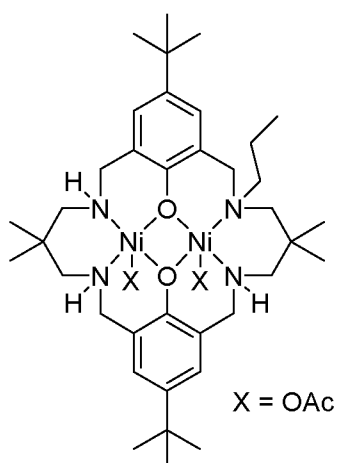
L^3Ni_2(OAc)_2
