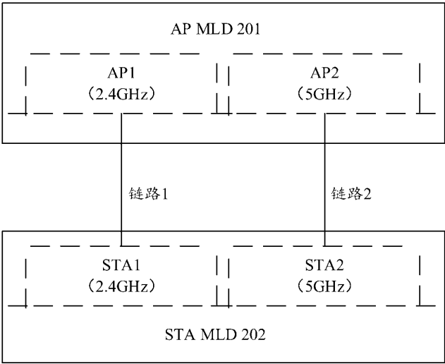
通信系统200
